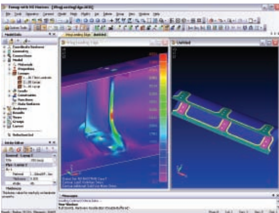
Visualizzazione di più viste dello stesso modello Femap e/o di più modelli nella stessa sessione di lavoro.
